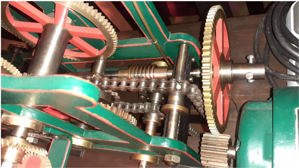
Abbildung 550: Turmuhr, Nebenuhr Schneckengetriebe
