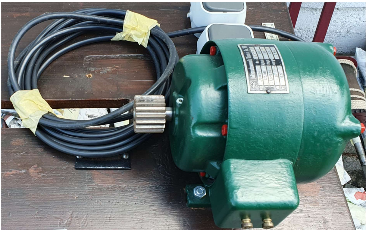
Abbildung 551: Turmuhr, Nebenuhr, Antriebsmotor
