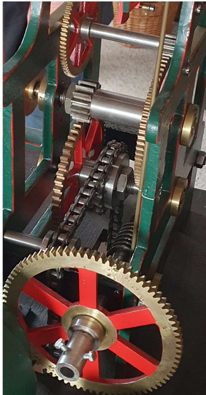
Abbildung 548: Turmuhr, Nebenuhr, Antrieb für Aufzug
