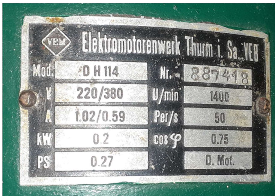
Abbildung 552: Turmuhr, Nebenuhr, Typschild Antriebsmotor
