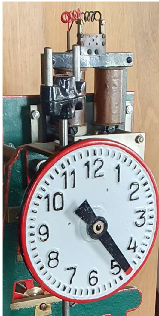
Abbildung 546: Turmuhr, Nebenuhr, Auslösung Nebenuhr, Kontrollzifferblatt mit Minutenanzeige
