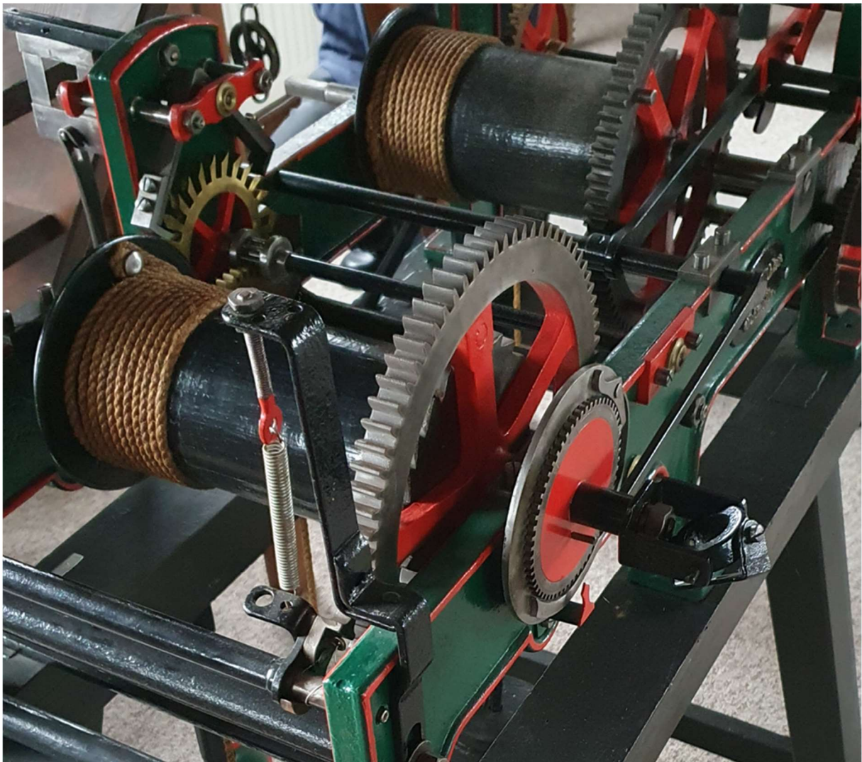
Abbildung 455: Turmuhr Jähler, Ansicht hinten links oben
