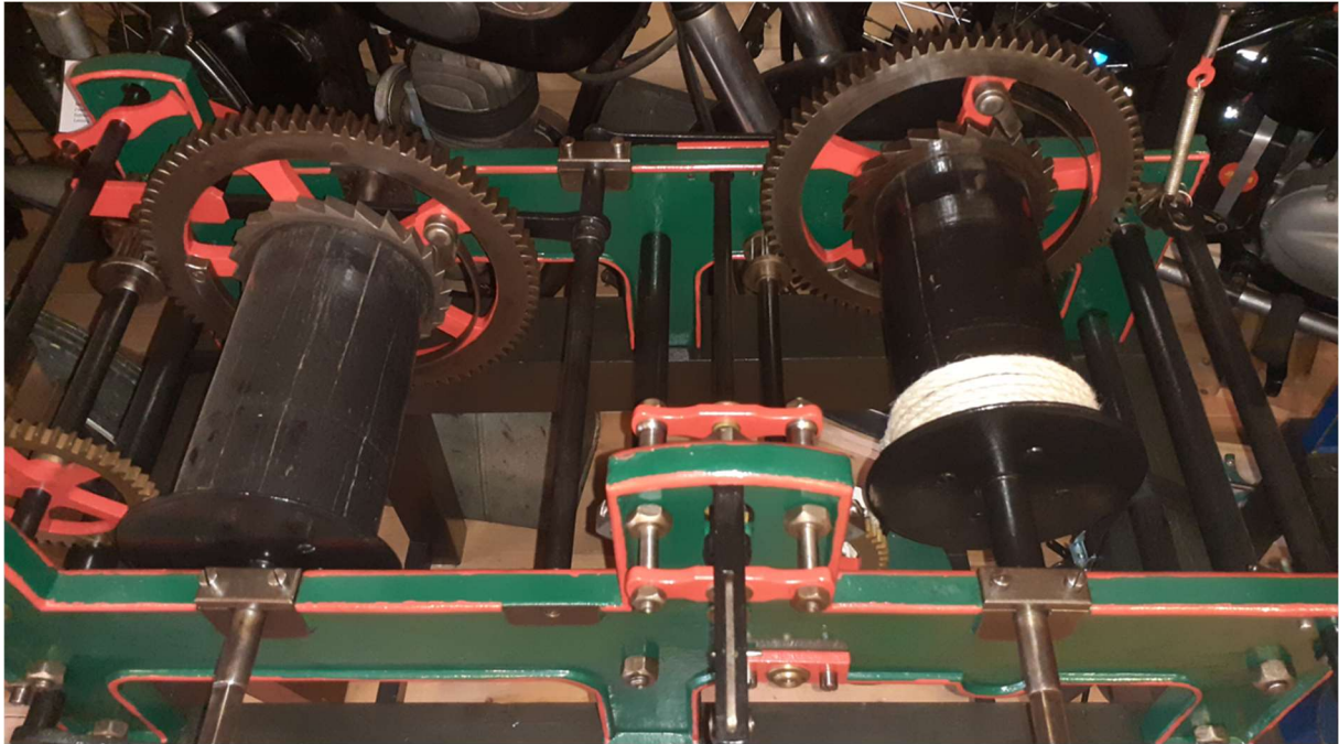
Abbildung 453: Turmuhr Jähler, Ansicht vorne oben
