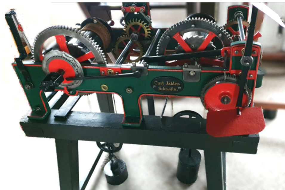
Abbildung 451: Turmuhr Jähler, Ansicht vorne oben
