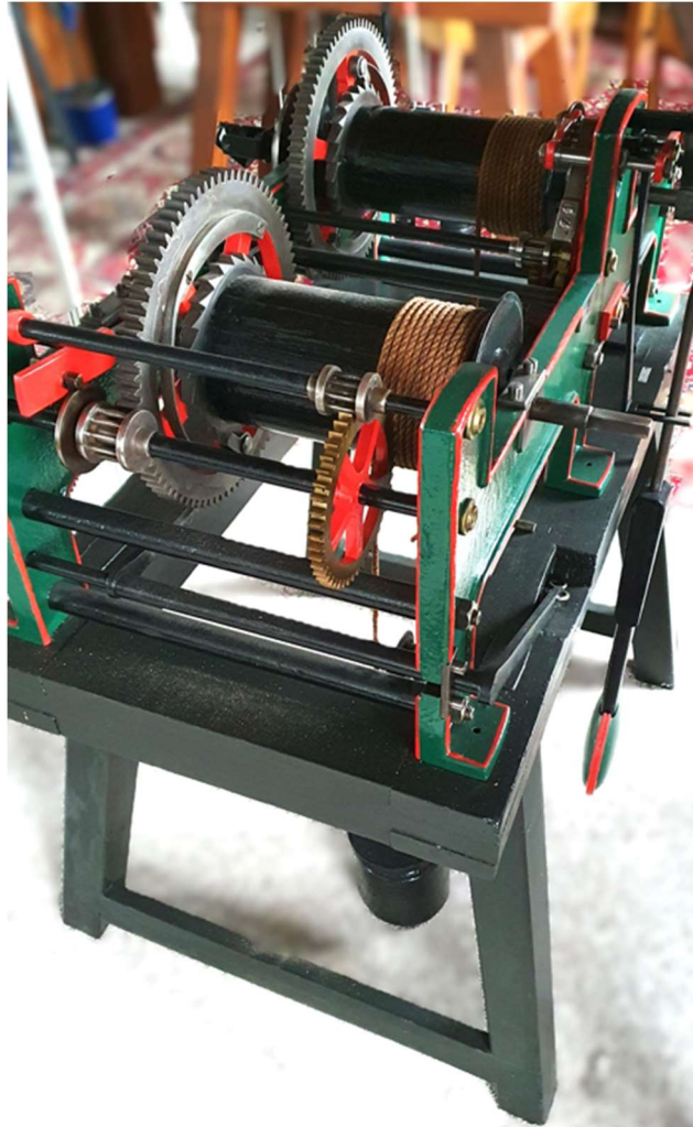
Abbildung 452: Turmuhr Jähler, Ansicht vorne links oben
