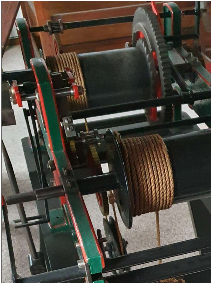
Abbildung 454: Turmuhr Jähler, Ansicht vorne rechts oben
