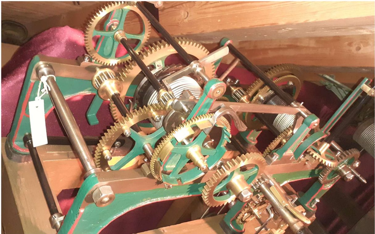
Abbildung 304: Turmuhr Zachariä, Ansicht vorne oben
