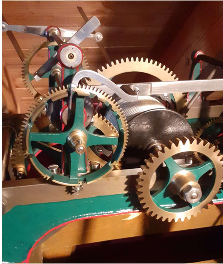
Abbildung 308: Turmuhr Zachariä, Schlagwerk
