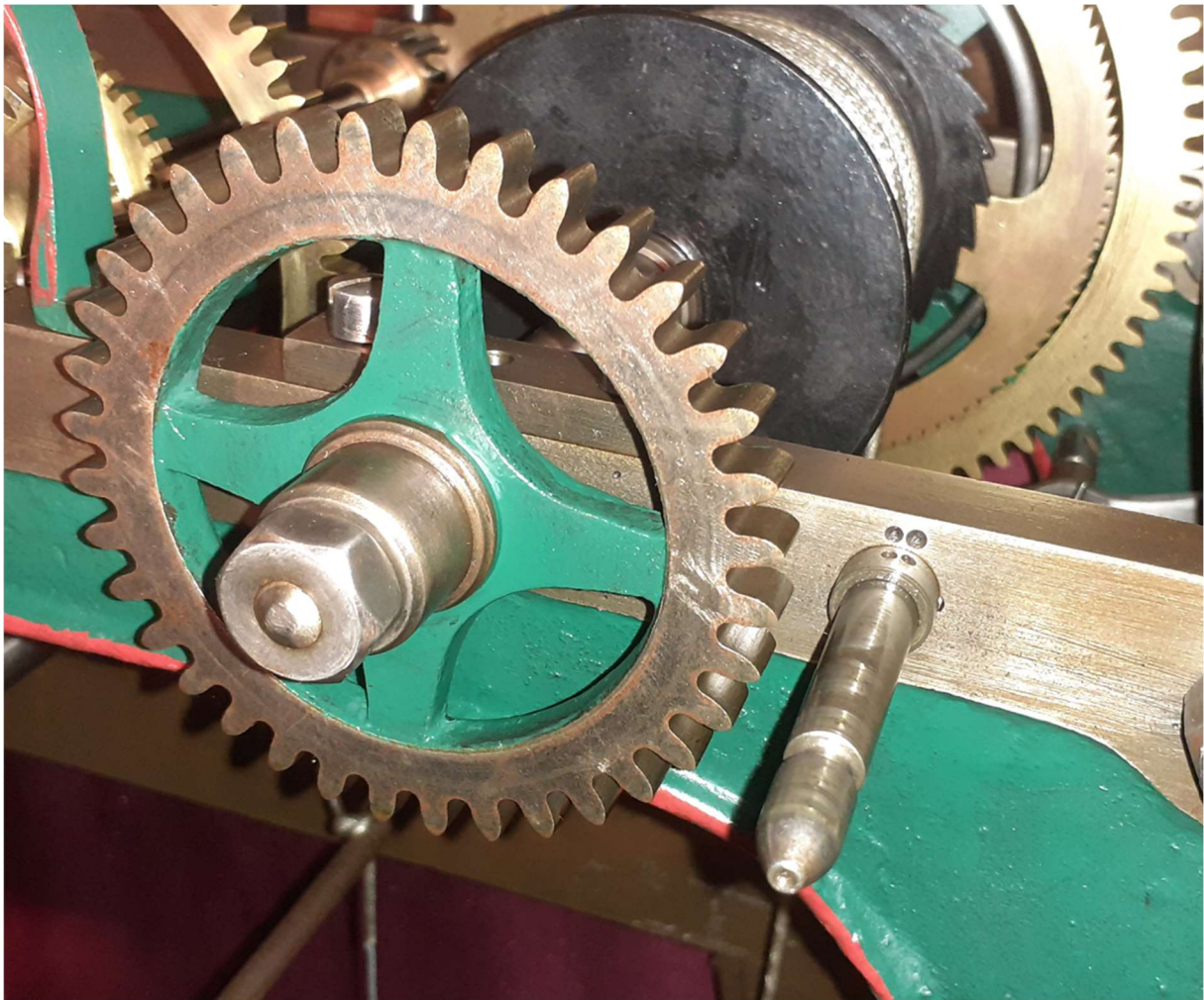
Abbildung 312: Turmuhr Zachariä, Aufzugseinrichtung Schlagwerk
