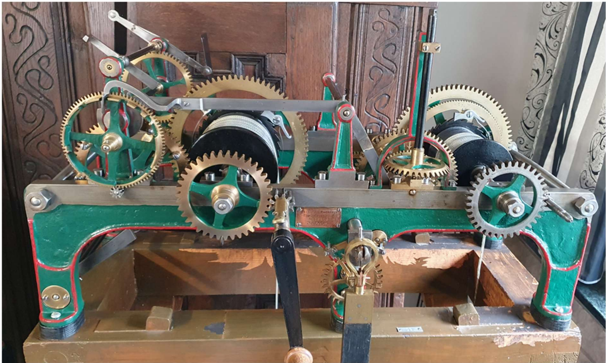
Abbildung 302: Turmuhr Zachariä, Uhrwerk vorne
