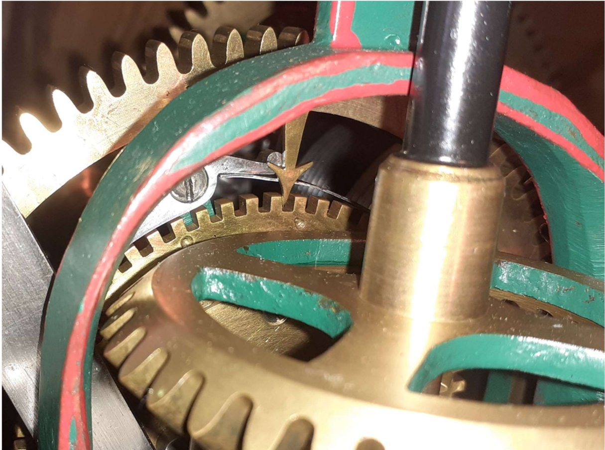
Abbildung 310: Turmuhr Zachariä, Pfeilzeiger für Minutenanzeige
