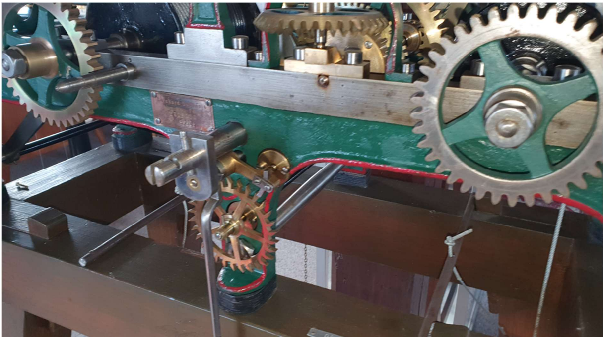
Abbildung 303: Turmuhr Zachariä, Graham-Hemmung
