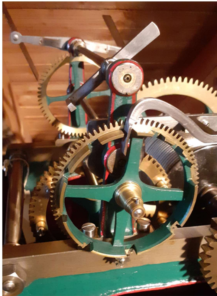
Abbildung 307: Turmuhr Zachariä, Schlagwerk, Schlossscheibe
