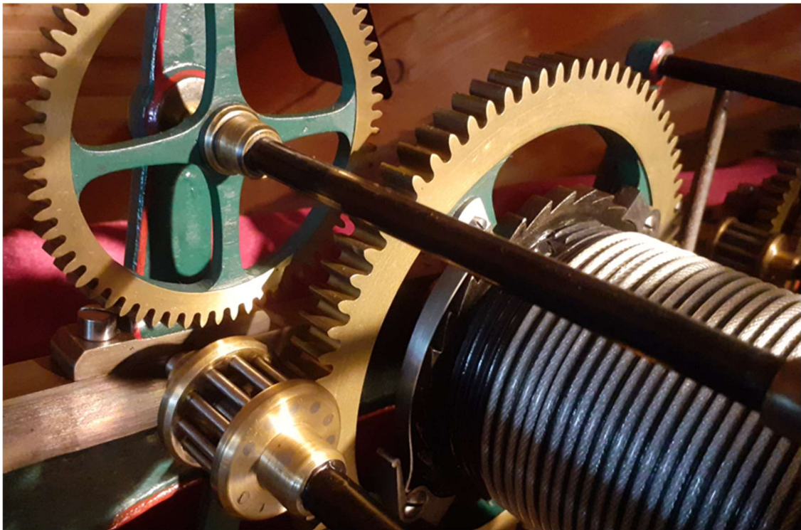
Abbildung 314: Turmuhr Zachariä, Getriebe
