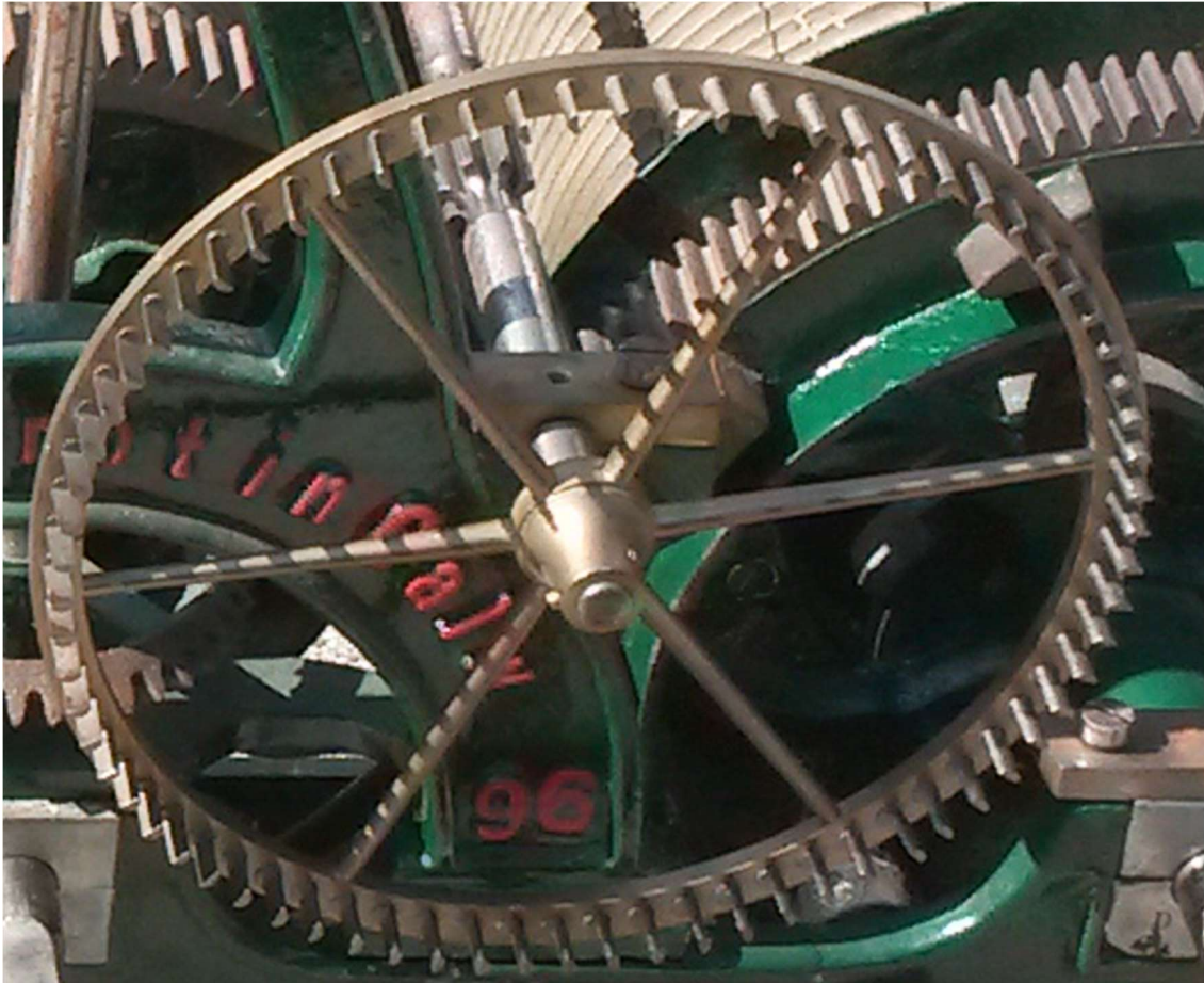
Abbildung 157: Turmuhr Perrot, Stiftenhemmung
