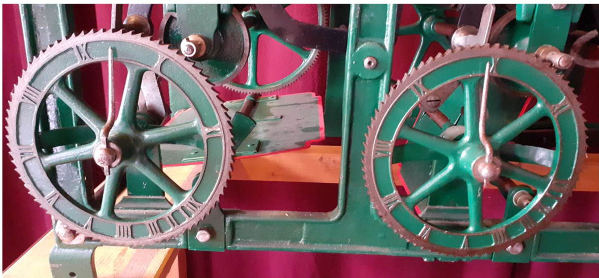
Abbildung 158: Turmuhr Perrot, Schlossscheiben
