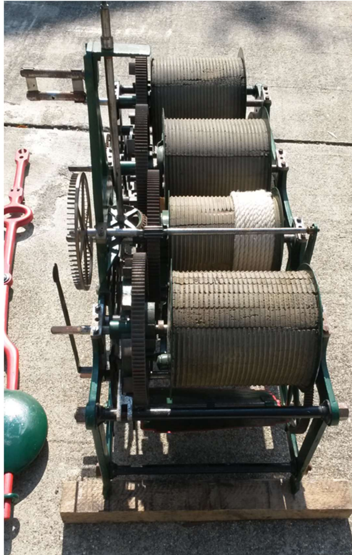
Abbildung 152: Turmuhr Perrot, Gesamtansicht rechts
