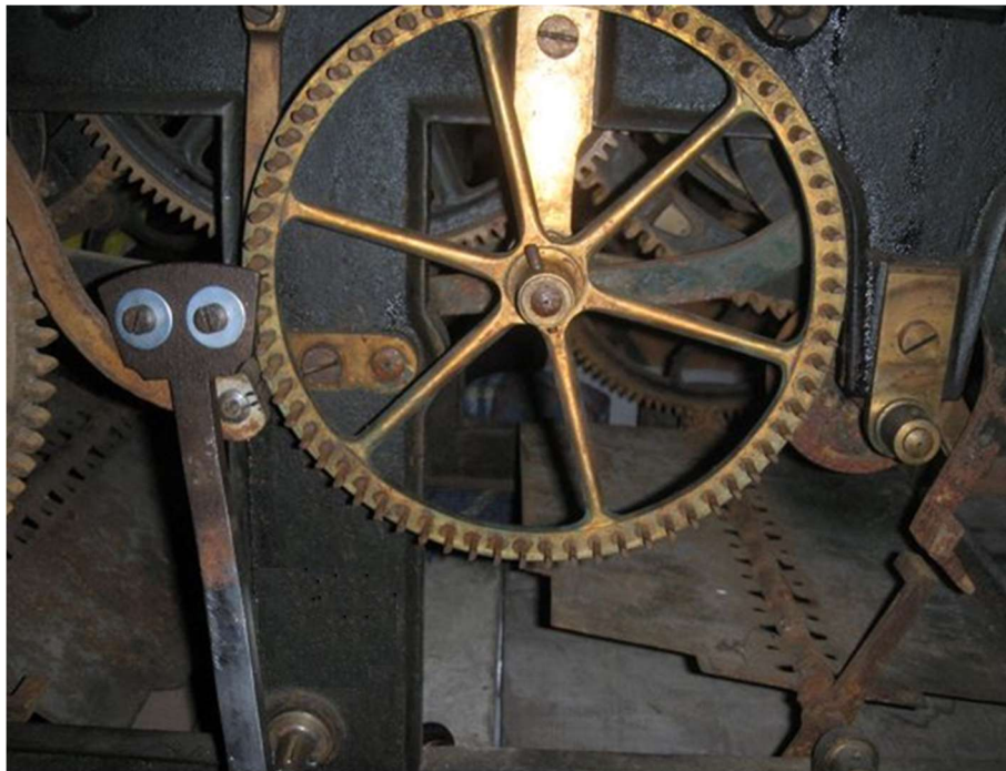
Abbildung 115: Turmuhr Mannhardt, Stiftenhemmung
