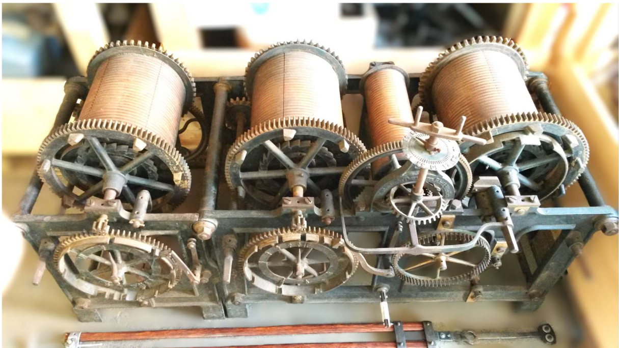
Abbildung 112: Turmuhr Mannhardt, Ansicht vorne oben
