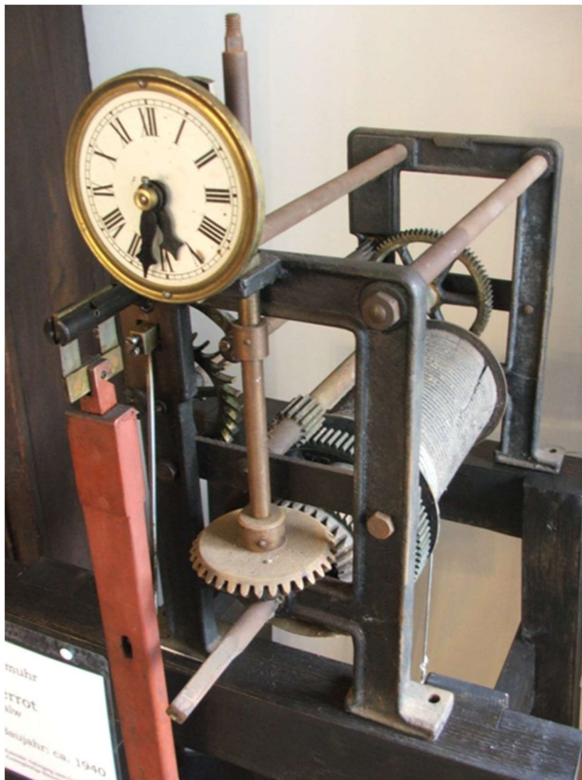
Abbildung 52: Turmuhr Perrot, Uhrwerk
