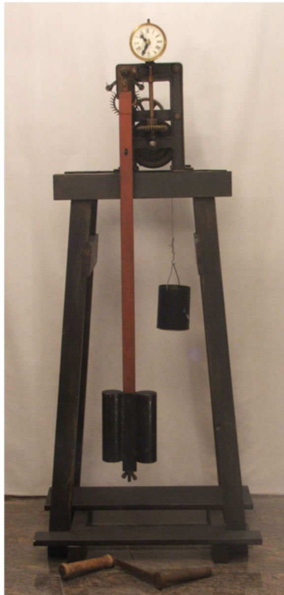
Abbildung 55: Turmuhr Perrot, Gesamtansicht
