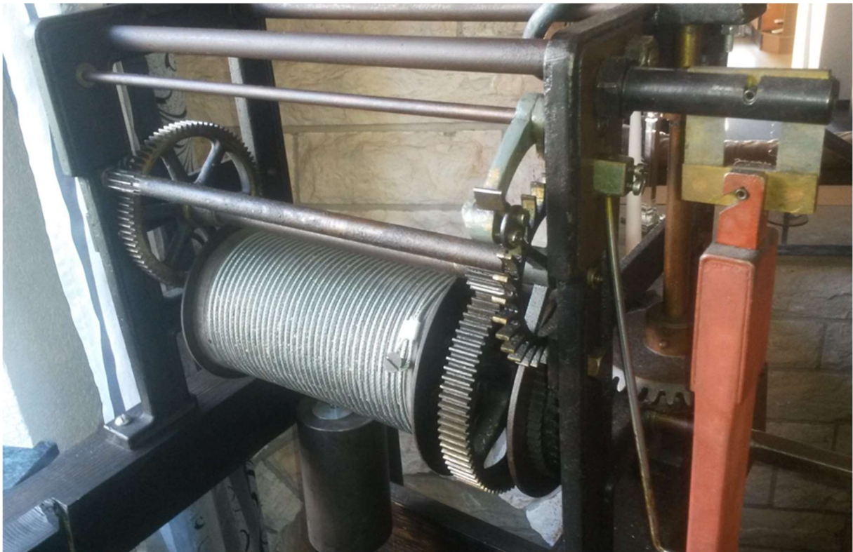
Abbildung 54: Turmuhr Perrot, Uhrwerk
