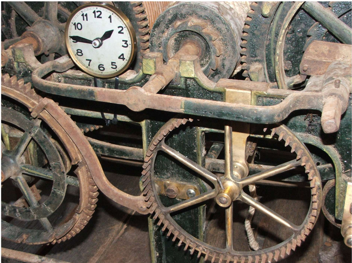
Abbildung 34: Turmuhr Neher und Söhne, Gehwerk
