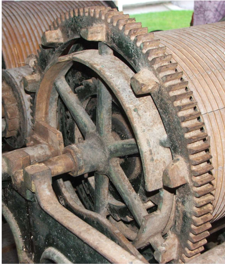
Abbildung 37: Turmuhr Neher und Söhne, Viertelstundenschlagwerk
